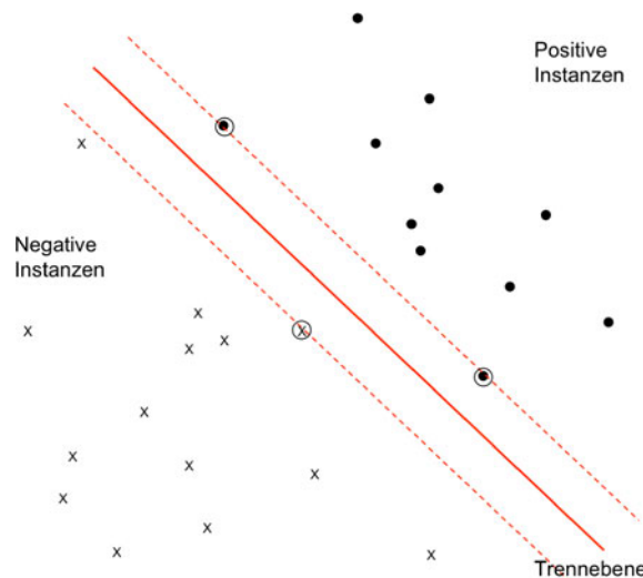
Abb. 3 Schematische Darstellung der Klassifikation mit Supportvektormaschinen. Die zu klassifizierenden Objekte sind durch ihre (hier zweidimensionalen) Merkmalsvektoren repräsentiert. Die Trennebene des Klassifikators wird so gewählt, dass sie die Vertreter beider Klassen (positive und negative Instanzen – Kreise und Kreuze) korrekt trennt und dabei die Trennbreite maximiert. Die Lage der Trennebene wird nur durch wenige Datenpunkte bestimmt, den Supportvektoren (markiert durch Ringe)
