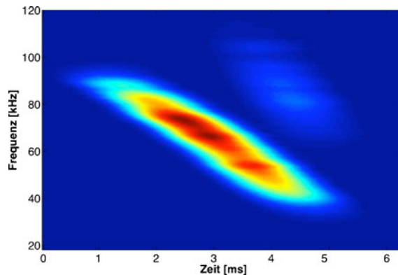
Abb. 5 Spektrogramm eines Echoortungslautes des großen Mausohrs ( Myotis myotis ). Die einfache Frequenz-Zeit-Struktur ist stark stereotypisiert und variiert nur wenig von Individuum zu Individuum, aber dafür umso stärker von Situation zu Situation
